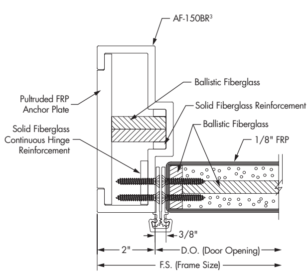
Hinge Jamb
