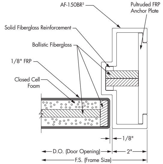
Lock Jamb
