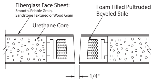
Optional Dual Bevel Stiles
