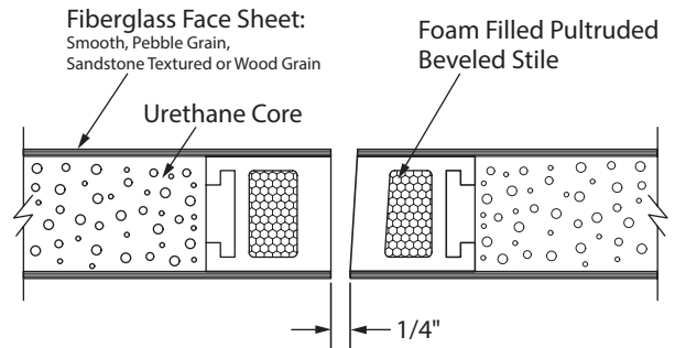
Standard Beveled Edge Lock Stile
