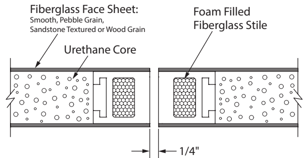
Optional Square Edge Lock Stile
