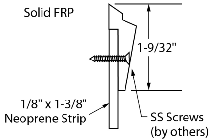
FRP Door Sweep
