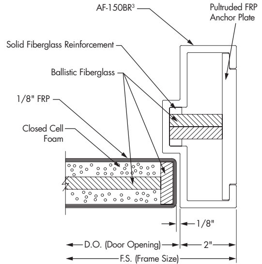
Lock Jamb
