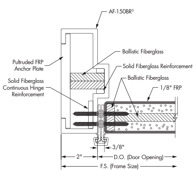
Hinge Jamb
