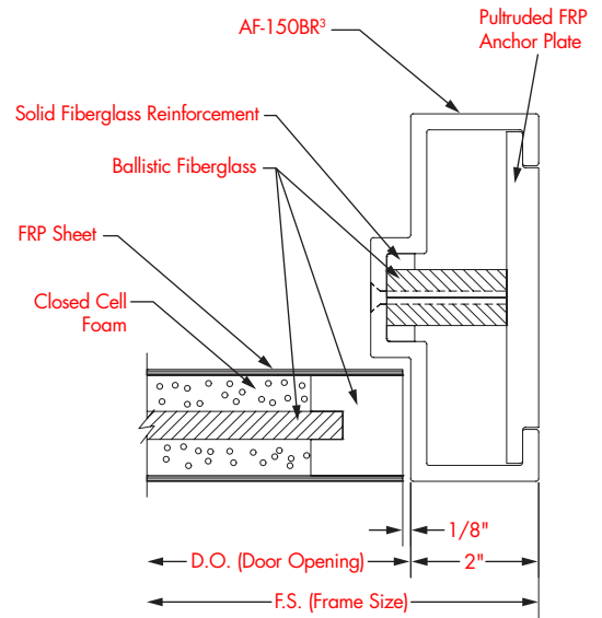
Lock Jamb
