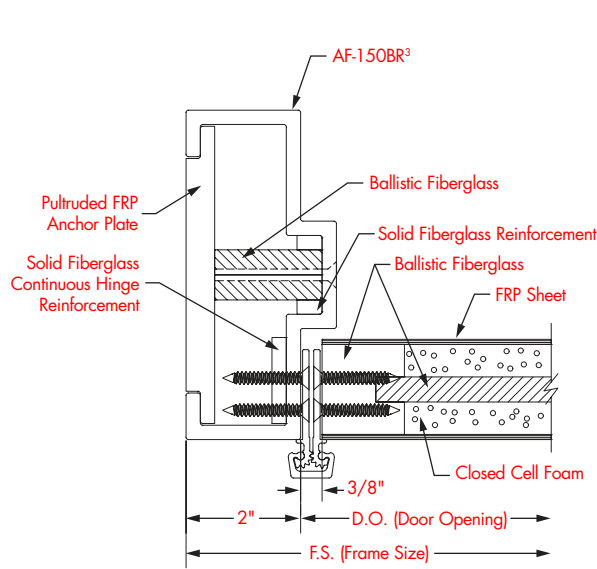
Hinge Jamb
