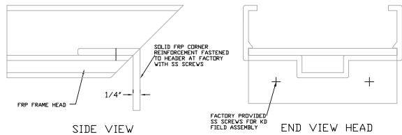
TYP CORNER REINFORCEMENT
