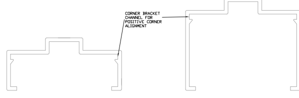
4" HEAD OPTIONAL
