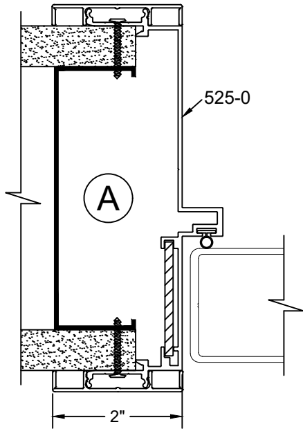
DOOR JAMB
