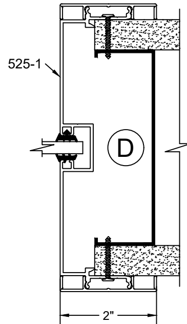
GLASS JAMB
