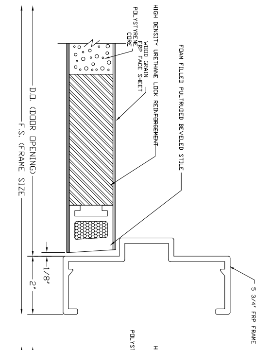
3 LOCK JAMB DETAIL 1:1
